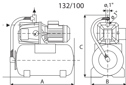
AQUAJET 102/-60-80 132/100
